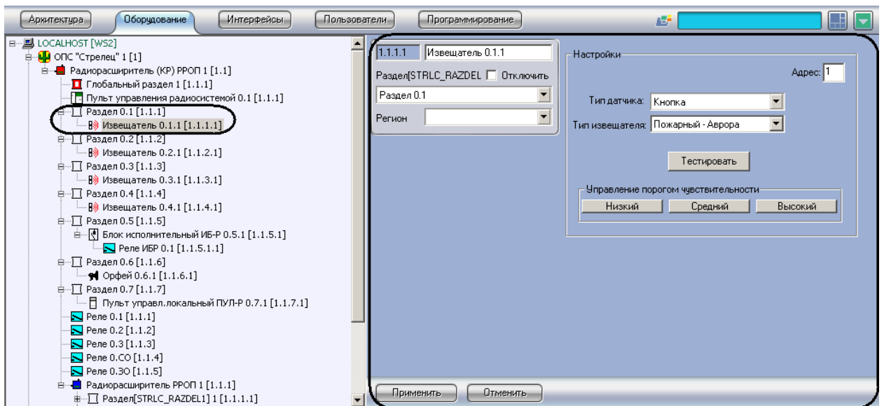
Рис. 3.4-1 Объект Извещатель
