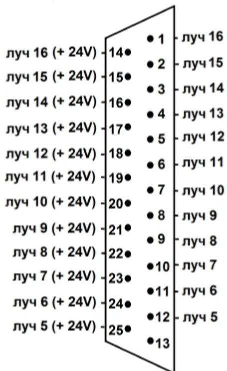
Разводка внешнего разъема интерфейсного кабеля лучи-реле
