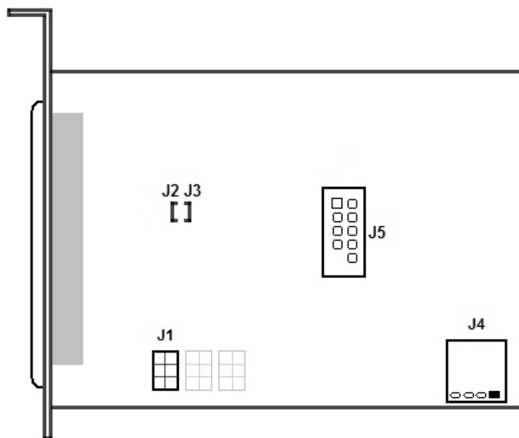
Схема разъемов платы SL USBIO:
