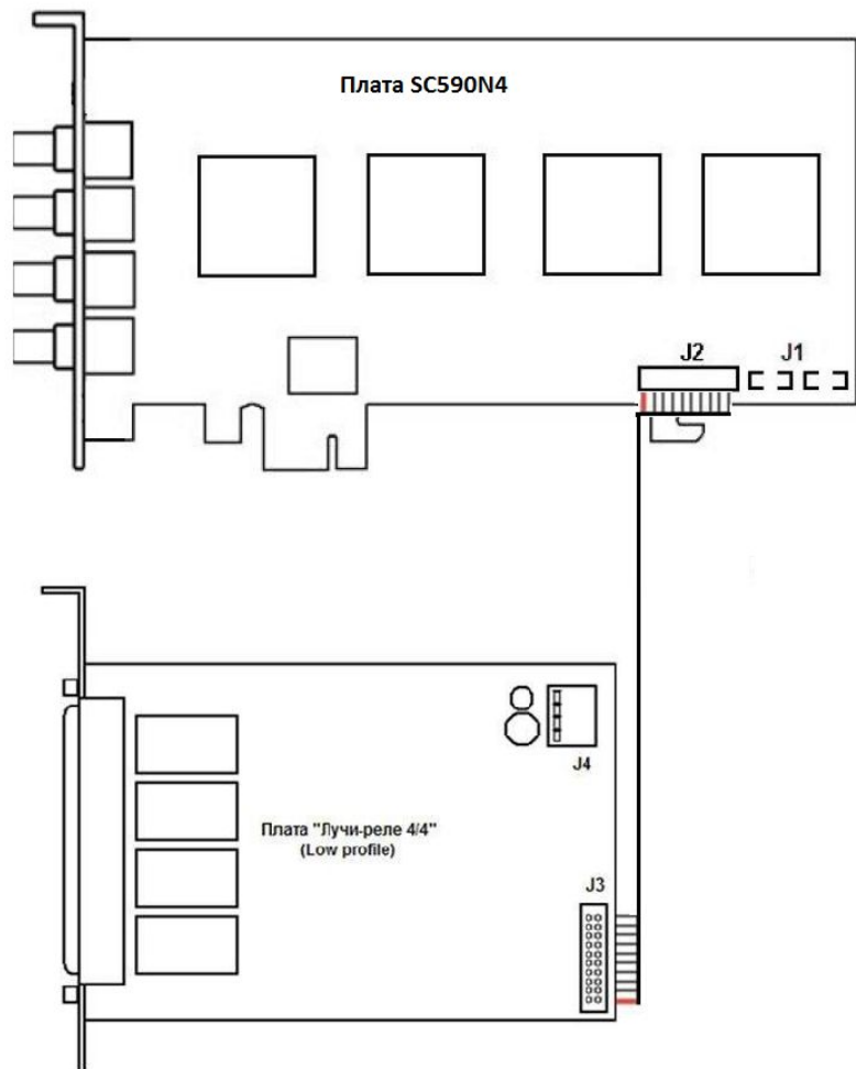
Схема подключения платы лучи-реле 4/4 (low profile) к плате SC590N4
