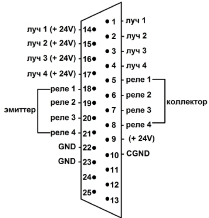
Разводка внешнего разъема интерфейсного кабеля лучи-реле
