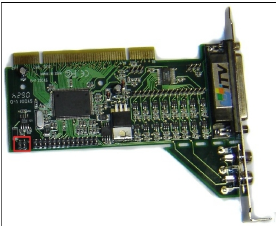
Два двухштырьковых разъема для подключения аппаратного контроля зависания Watchdog (на примере платы видеоввода SC300Q16 (FX4)):
