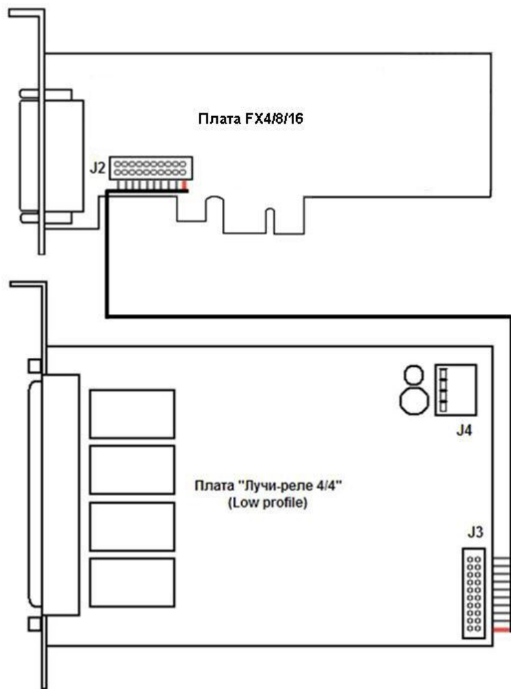
Схема подключения платы лучи-реле 4/4 (low profile) к платам SC300Q16, SC300D16, SC310N16 (FX4/8/16)
