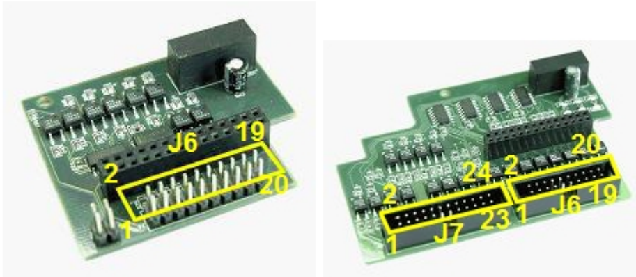
Разъемы на плате лучи-реле для подключения интерфейсного кабеля (на примере плат лучи-реле 4/4 и 16/4)
