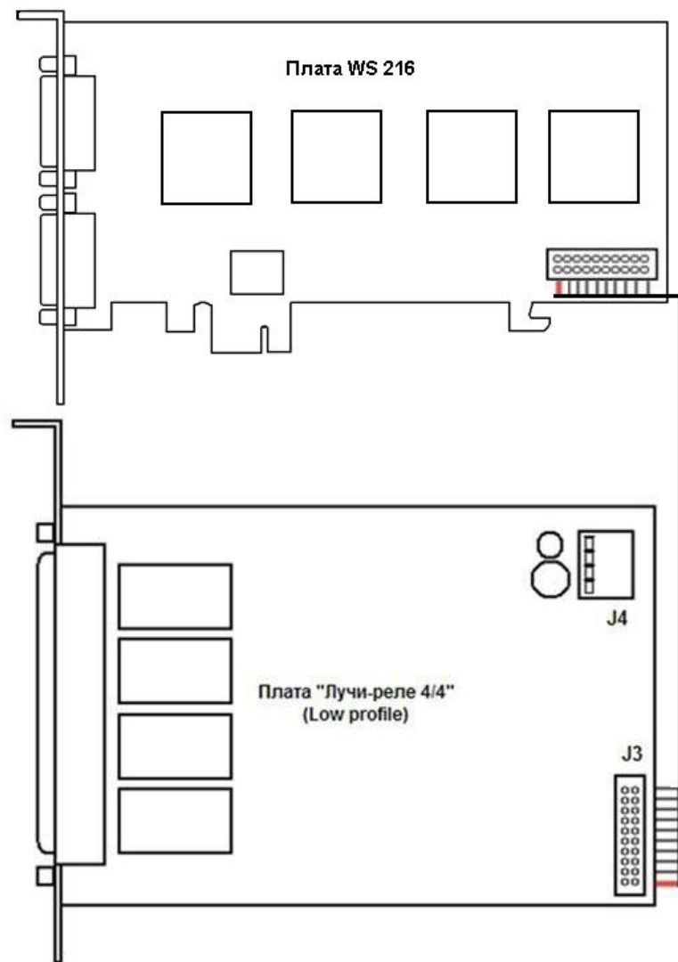
Схема подключения платы лучи-реле 4/4 (low profile) к плате SC3B0N16 (WS216)
