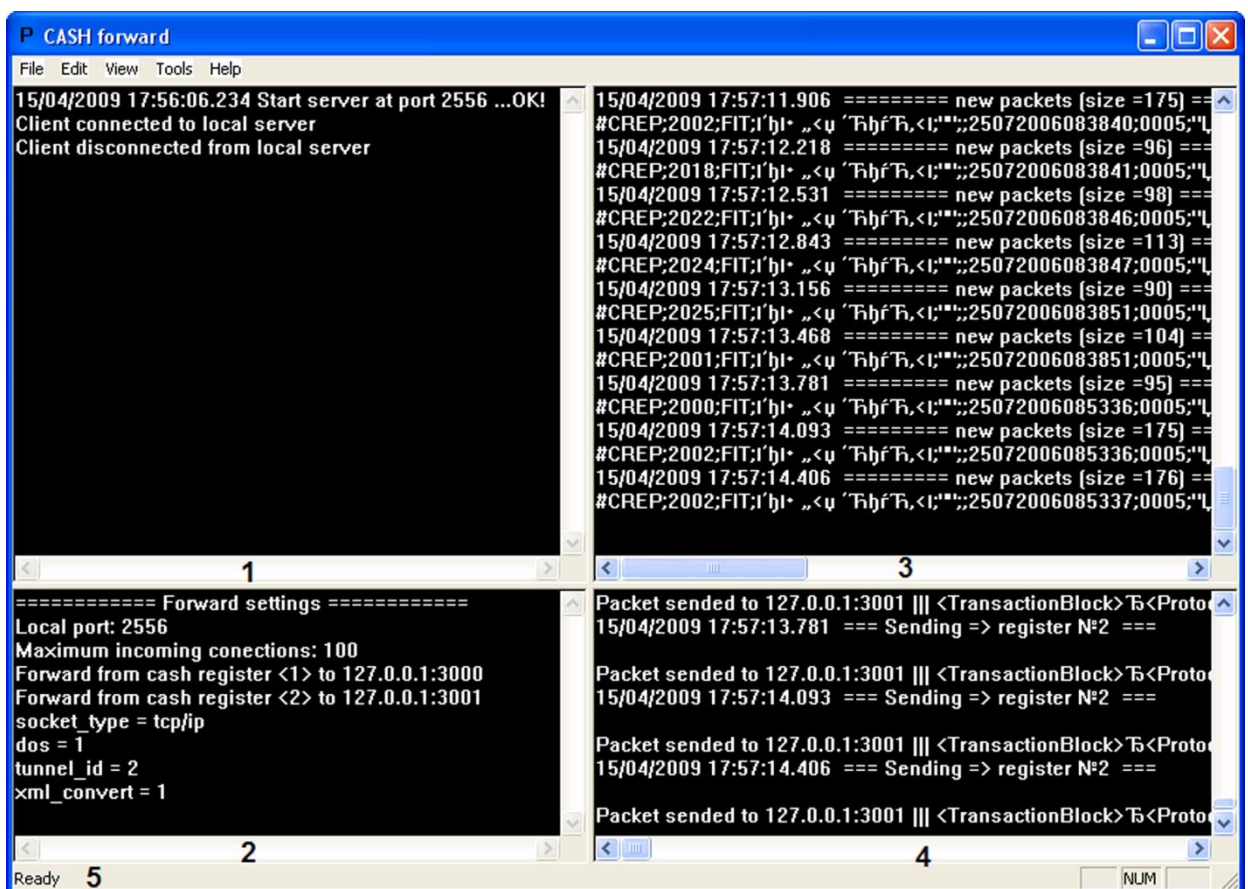
Рис. 11.3—1. Окно утилиты «CASH forward»
