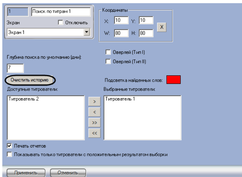
Рис. 6.4—13. Очистка истории пользовательских запросов
