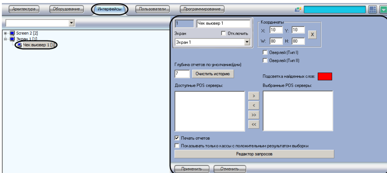
Рис. 6.5—1. Настройка интерфейсного объекта «Чек выювер»
