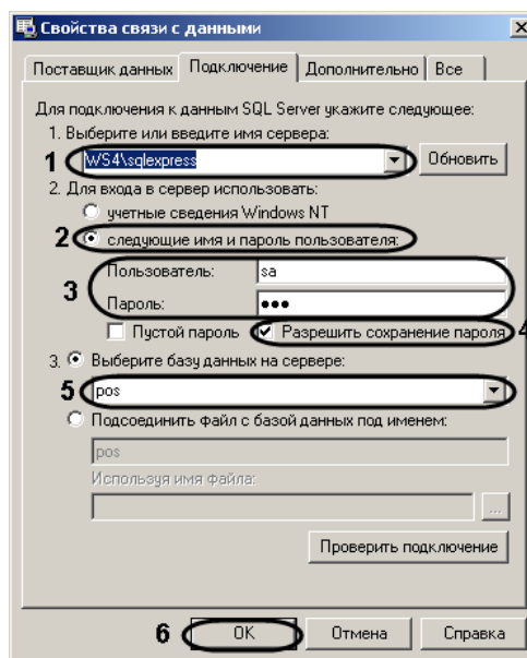
Рис. 6.7—3 Настройка подключения к базе данных
