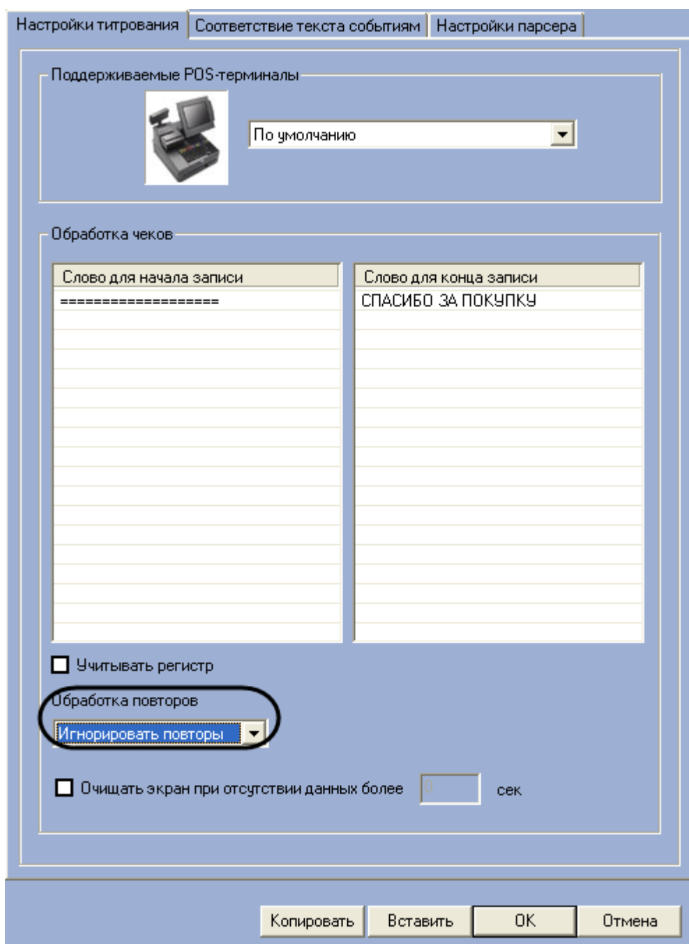
Рис. 6.3—13. Задание обработки повторов
