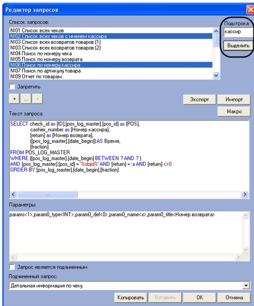
Рис. 6.5—25. Поиск в списке «Список запросов» заданной подстроки
