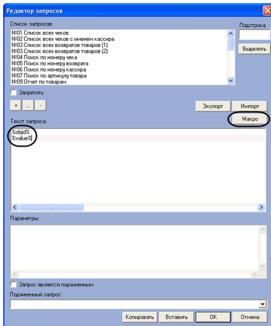
Рис. 6.5—24. Доступ к шаблонным компонентам языка SQL
