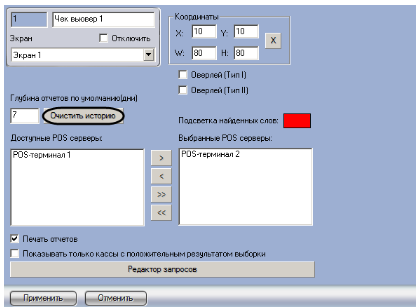
Рис. 6.5—13. Очистка истории пользовательских запросов
