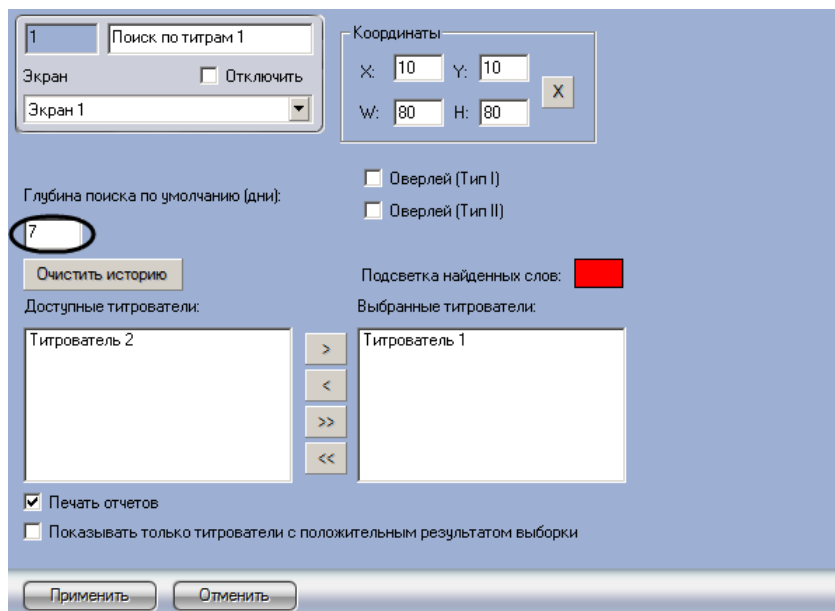
Рис. 6.4—5. Задание глубины поиска по базе данных титров
