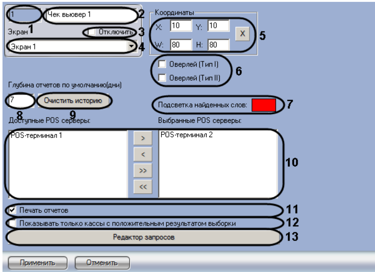
Рис. 7.4—1. Панель настройки интерфейсного объекта «Чек вьювер»
