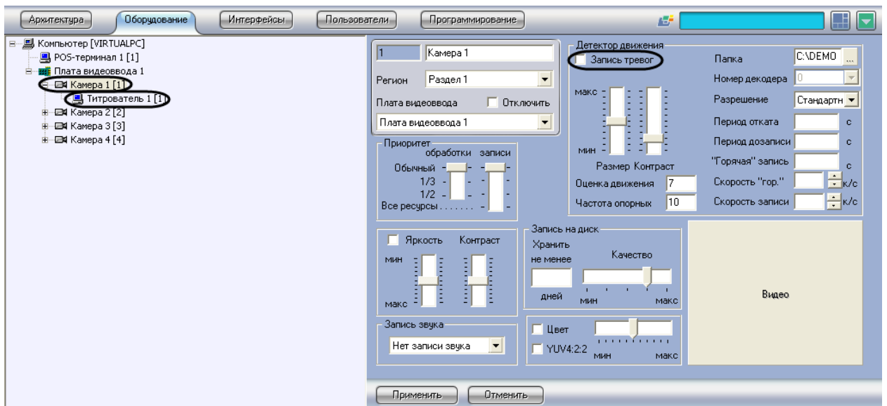
Рис. 6.3—21. Опция «Запись тревог» (объект «Камера»)
