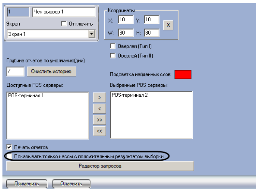
Рис. 6.5—8. Опция «Показывать только кассы с положительным результатом выборки»
