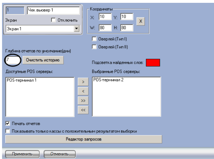
Рис. 6.5—5. Задание глубины поиска по базе данных чеков
