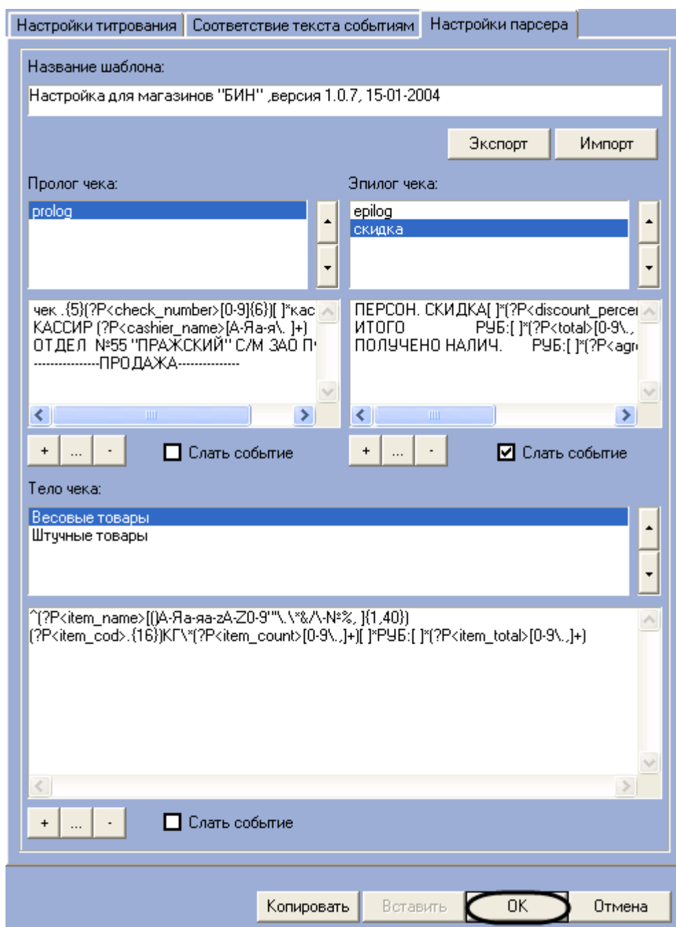
Рис. 6.3—49. Закрытие диалогового окна "Дополнительно"
