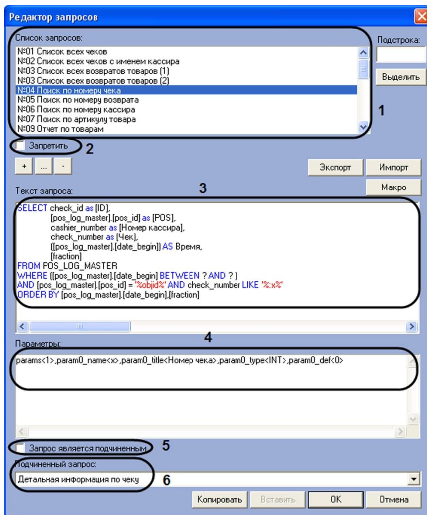
Рис. 6.5—23. Отображение параметров пользовательского запроса
