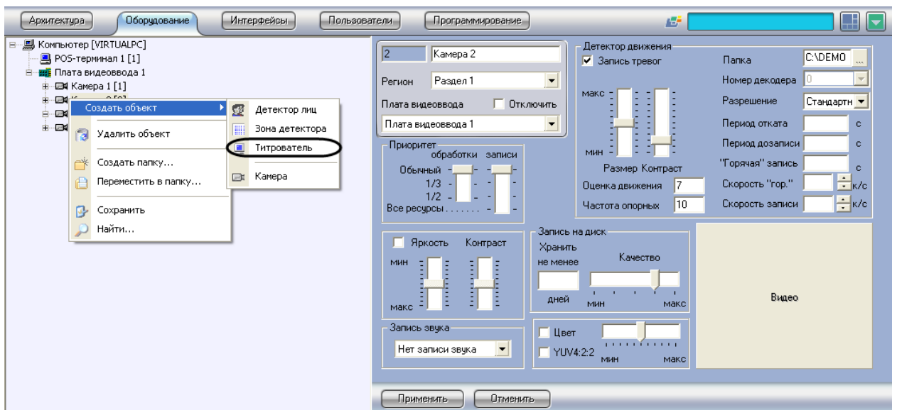
Рис. 6.2—2. Контекстное меню объекта «Камера»
