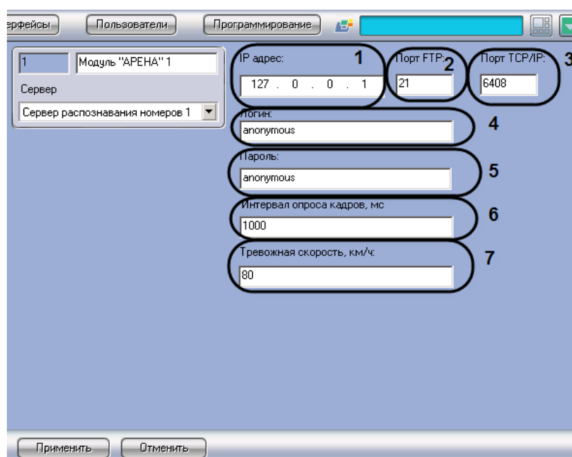
Рис. 8.11—1 Панель настроек объекта «Модуль «Арена»»
