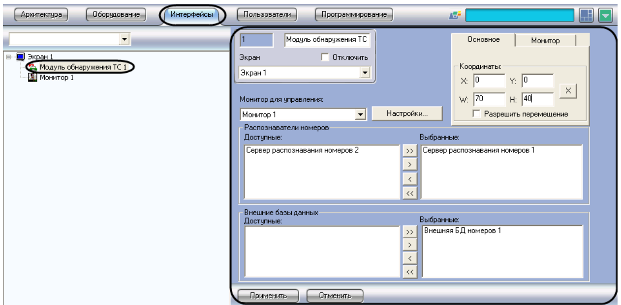
Рис. 7.8—1. Объект «Модуль обнаружения ТС»
