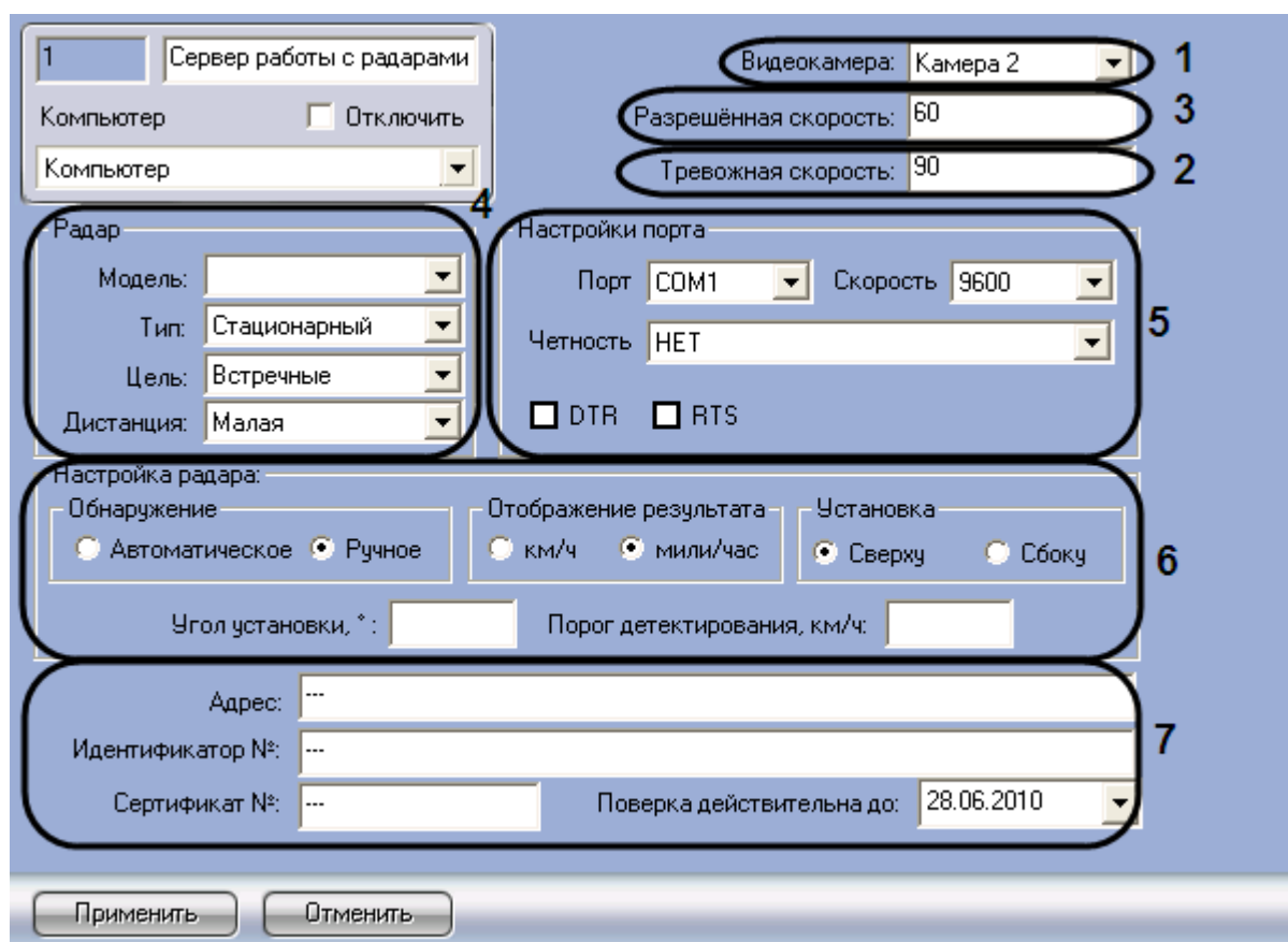
Рис. 8.2—1. Панель настройки объекта «Сервер работы с радарамии»
