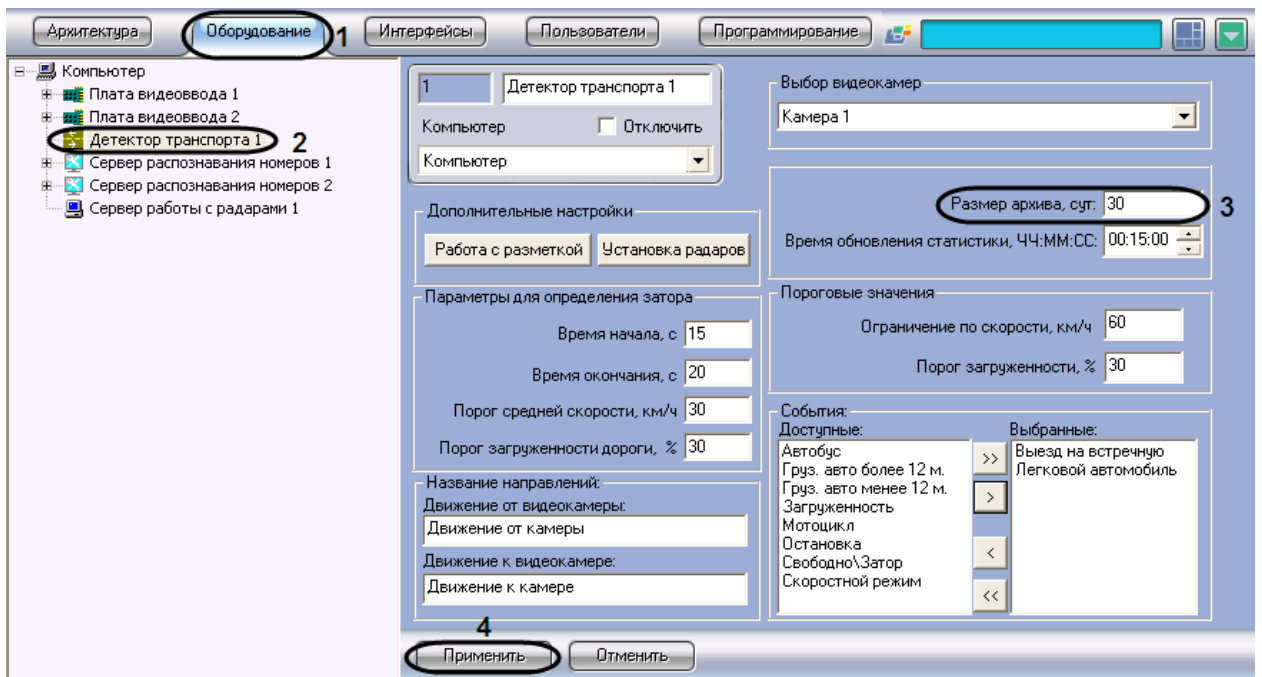
Рис. 7.4—2. Настройка глубины хранения записей в базе данных
