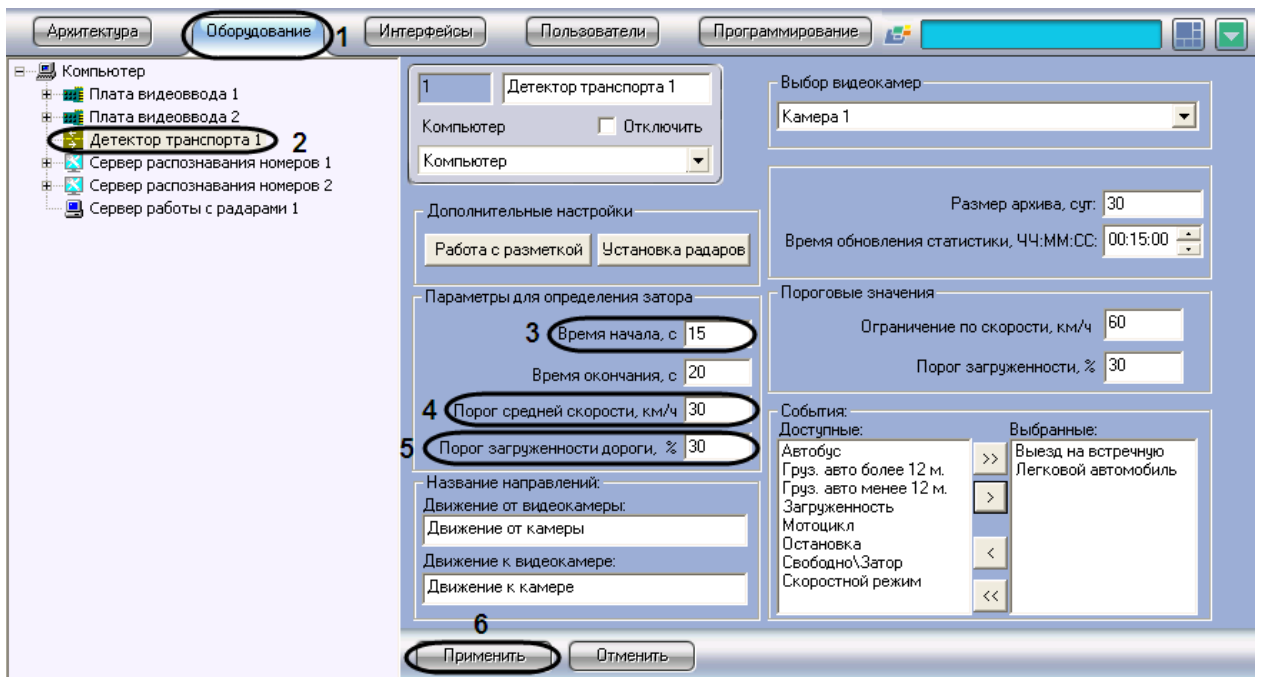
Рис. 7.4—17. Указание параметров образования затора на дороге
